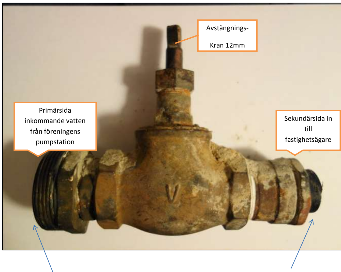
Servisventilens primärsida PEM-slang R 50
